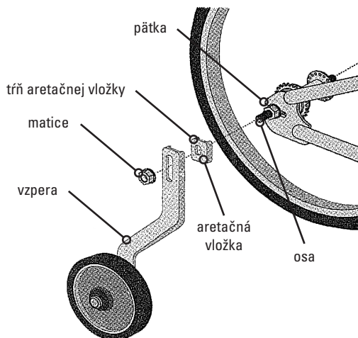
obrázok 31 - pomocné koliesko
