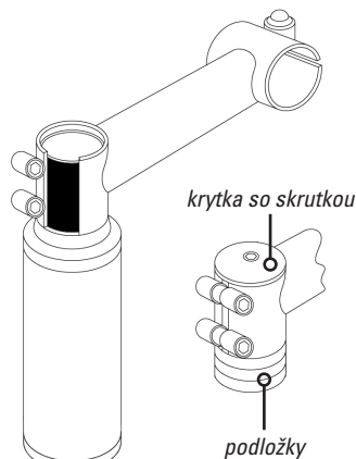
obrázok 5 - predstavca typu A-head
