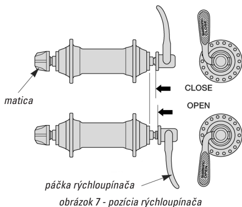
obrázok 7 - pozícia rýchlopínača
