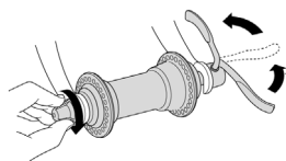
obrázek 8 - nastavení matice
