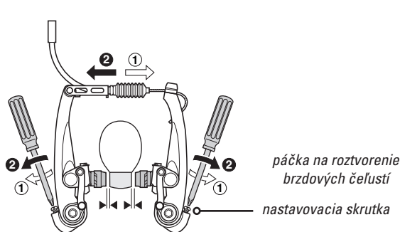
obrázok 15 - nastavenie brzdy typu V
