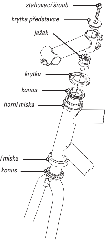
obrázek 27 - hlavové složení pro bezzávítovou vidlici
