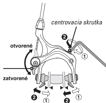
obrázok 16 - nastavenie cestnej brzdy
