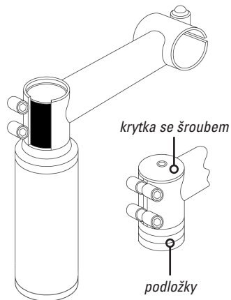
obrázek 5 - představec pro bezzávitovou vidlici
