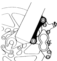
obrázek 13 - kotoučová brzdá
